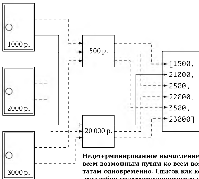
Рис. 29.4: Список как недетерминированное вычисление
