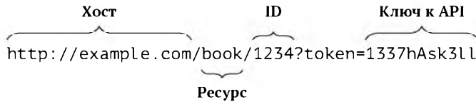
Рис. 5.3: Составные части URL
