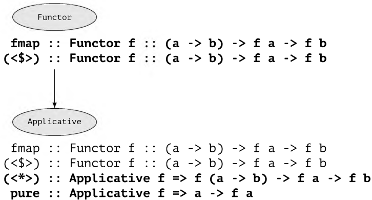
Рис. 29.1: Класс типов Functor является родительским для Applicative
