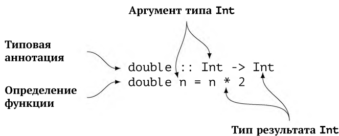
Рис. 11.2: Определение функции double с явным указанием типа
