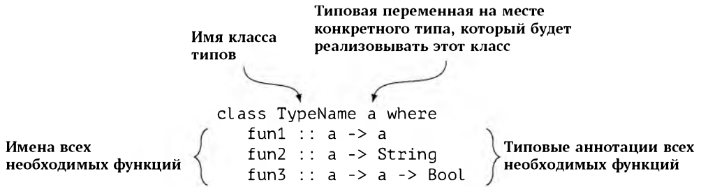
Рис. 13.1: Структура определения класса типов
