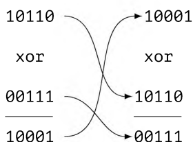
Рис. 15.2: Симметричная природа XOR
