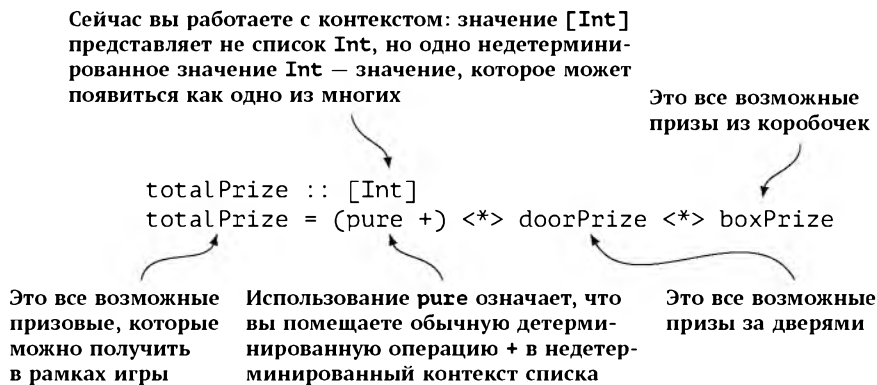
Рис. 29.5: Недетерминированное вычисление всех путей развития событий
