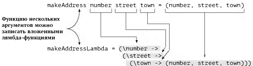
Рис. 11.4: Представление makeAddress в виде функции одного аргумента
