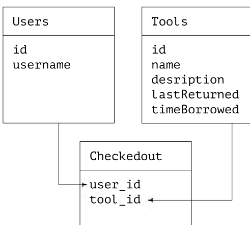
Рис. 41.1: Схема базы данных
