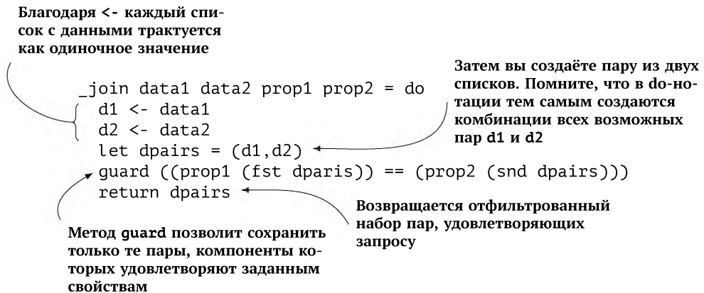
Рис. 33.5: _join соединяет два набора данных с совпадающими полями
