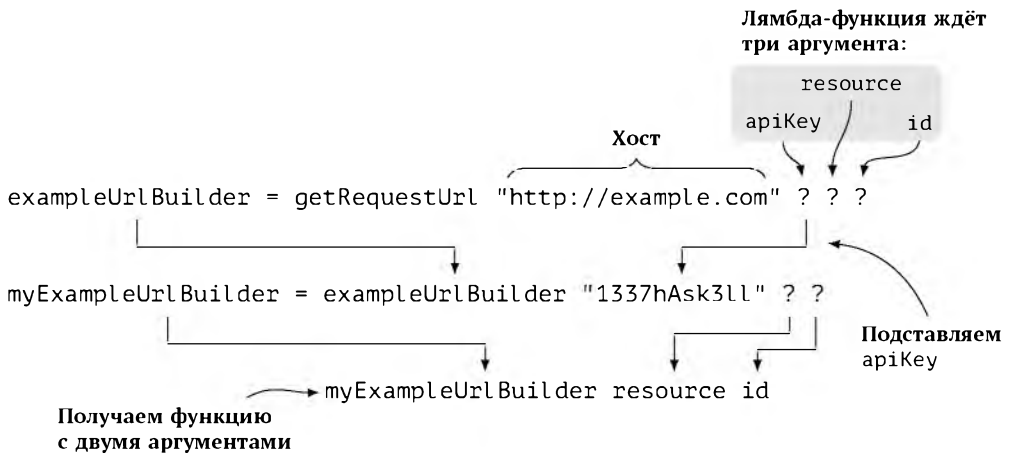
Рис. 5.5: Визуальное представление частичного применения функции
