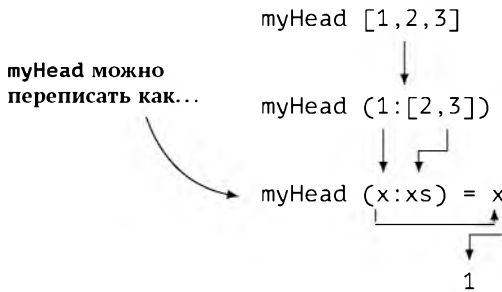
Рис. 7.1: Визуализация сопоставления с образцом в функции myHead
