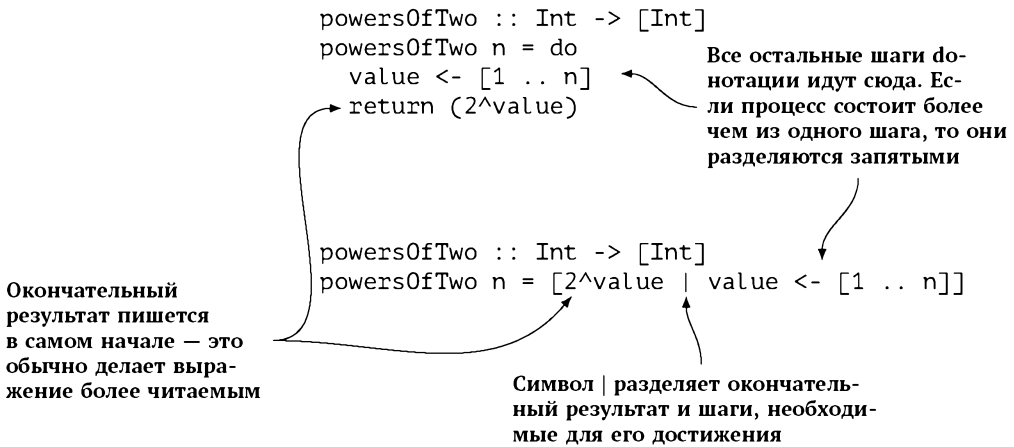
Рис. 32.2: Генераторы списков упрощают do-нотацию
