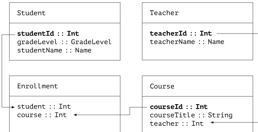
Рис. 33.1: Отношения между данными, с которыми мы будем работать
