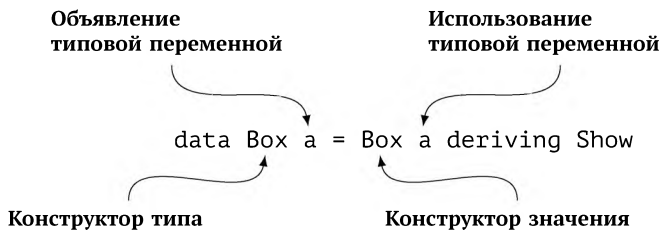
Рис. 18.1: Определение параметризованного типа Box
