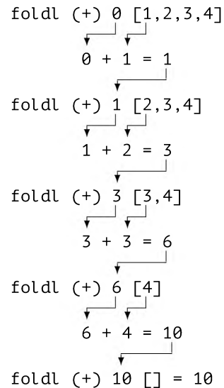
Рис. 9.1: Визуализация foldl (+)
