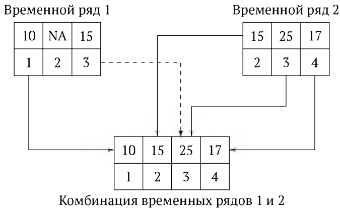
Рис. 20.2: Комбинирование двух временных рядов
