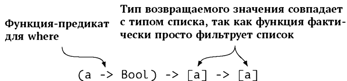
Рис. 33.3: Тип функции where
