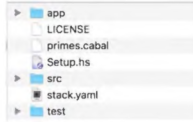
Рис. 37.1: Файлы, созданные утилитой stack
