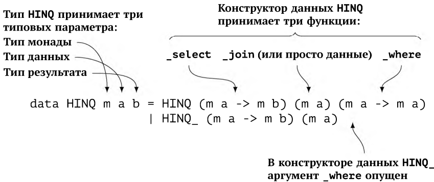
Рис. 33.6: Определение типа HINQ с комментариями
