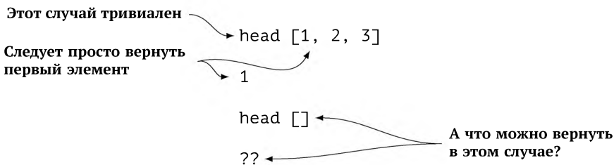
Рис. 38.1: Проблема с поведением head на пустом списке
