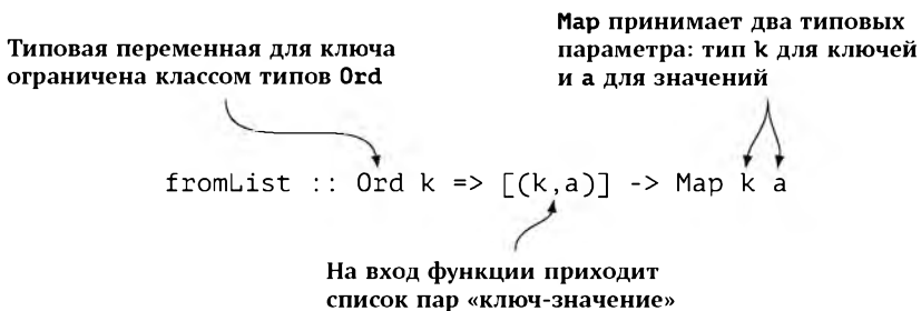
Рис. 18.4: Функция fromList для построения Map
