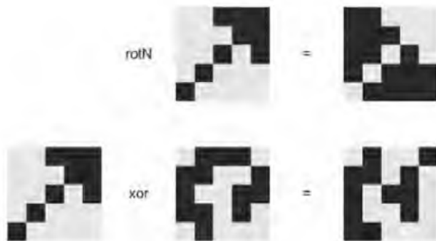
Рис. 15.3: Сравнение кодирования rotN и XOR на примере картинки
