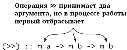
Рис. 30.6: Операция >> странного типа для монад с побочными эффектами
