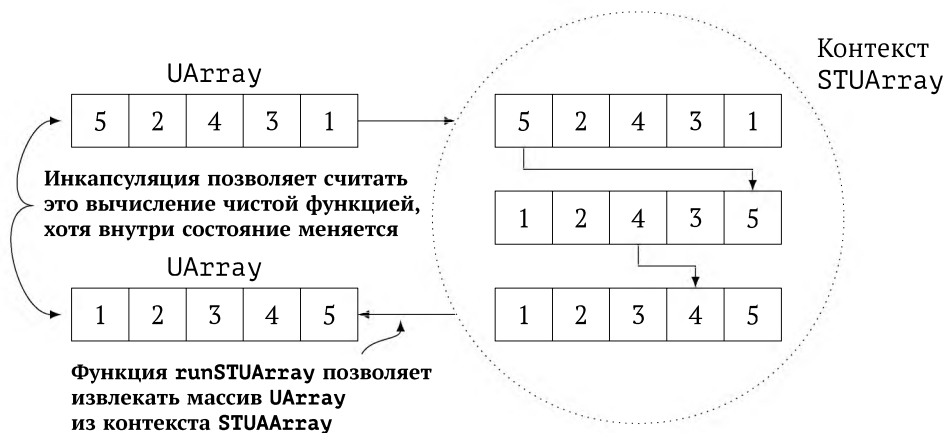
Рис. 42.2: Контекст STUArray поддерживает извлечение значений
