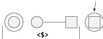
Рис. 27.2: Функция fmap (или <$> ) как адаптер и типы в контексте
