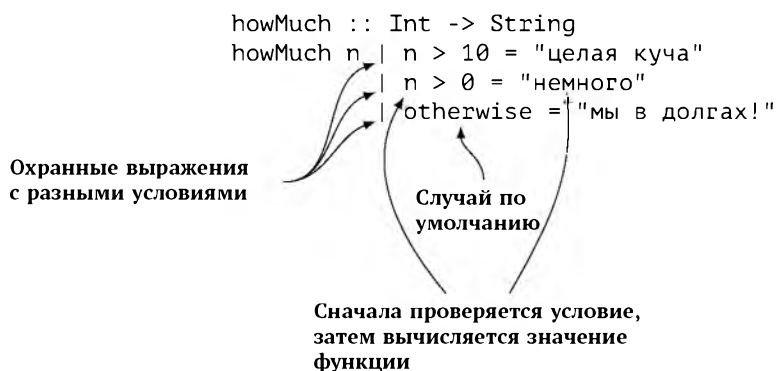
Рис. 17.1: Использование охранных выражений в функции howMuch
