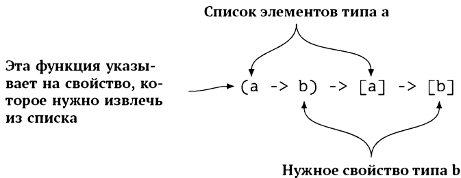
Рис. 33.2: Тип функции select
