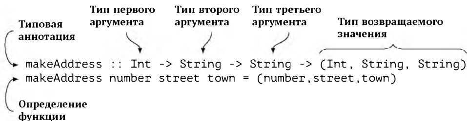
Рис. 11.3: Типовая аннотация и определение функции makeAddress
