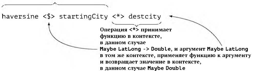
Рис. 28.5: Использование <$> и <*> для вычислений в контексте Maybe
