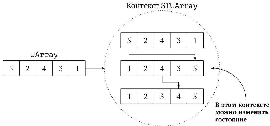
Рис. 42.1: Контекст STUArray с возможностью изменять состояние
