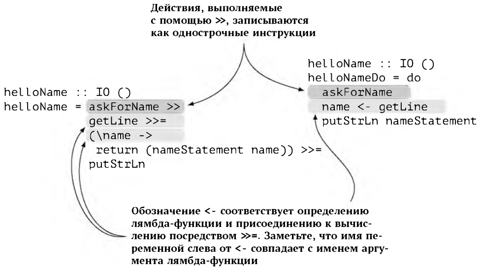
Рис. 31.1: Соответствие между методами класса Monad и do-нотацией
