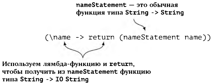
Рис. 30.7: Лямбда-функция для преобразования типа a -> a в a -> m a
