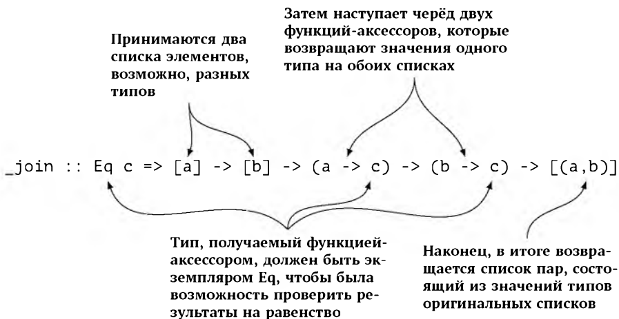
Рис. 33.4: Тип _join с пояснениями
