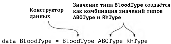
Рис. 12.2: Комбинирование ABOType и RhType для создания BloodType
