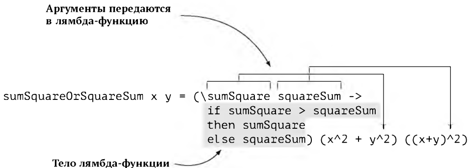
Рис. 3.2: Реализация sumSquareOrSquareSum через лямбда-функции
