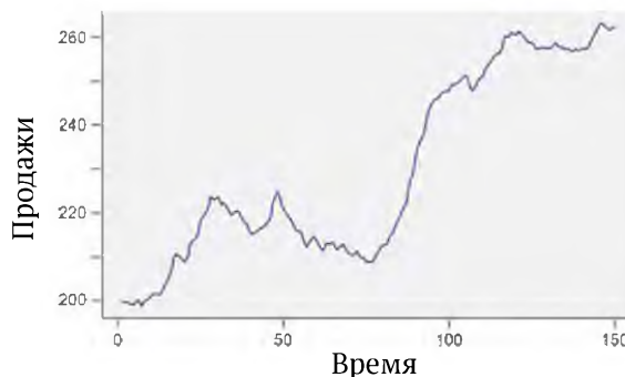
Рис. 20.1: Пример временного ряда продаж (Бокс и Дженкинс, 1976)
