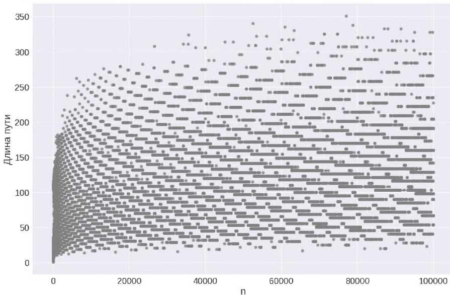
Рис. 8.1: Гипотеза Коллатца: длины путей до достижения единицы
