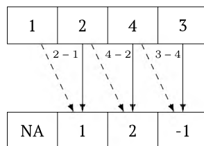
Рис. 20.3: Вычисление разностей
