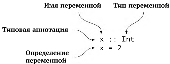
Рис. 11.1: Типовая аннотация
