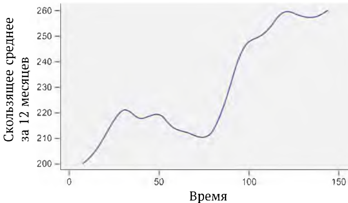
Рис. 20.5: Ряд, сглаженный скользящим средним по 12 месяцам
