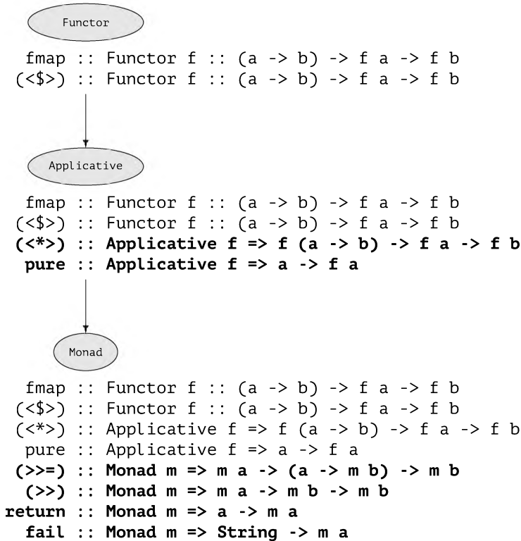
Рис. 30.5: Соотношение между классами Functor , Applicative и Monad
