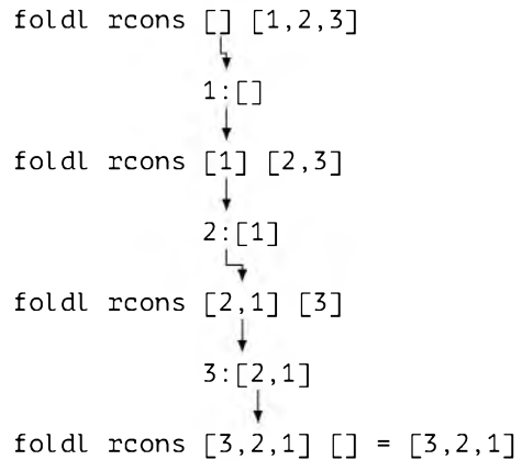
Рис. 9.2: Визуализация foldl rcons
