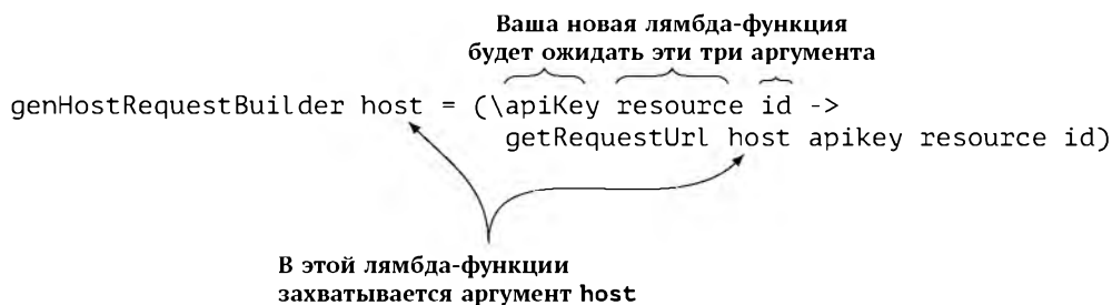
Рис. 5.4: Захват значения host в замыкании
